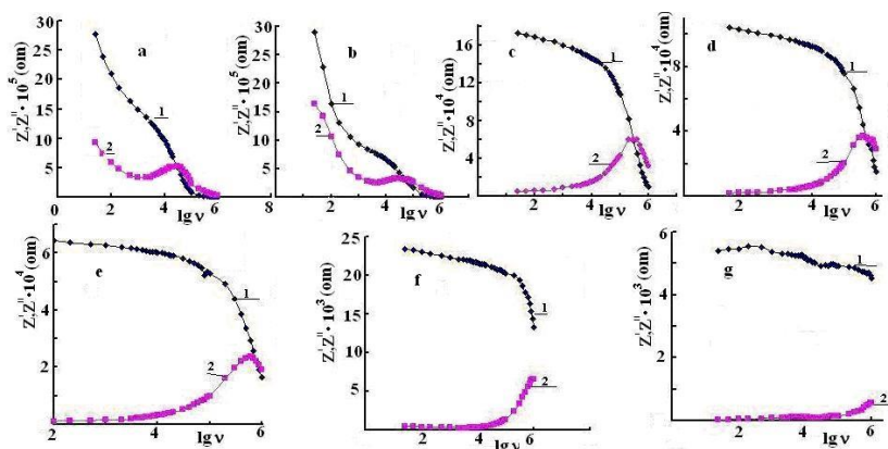
Рис.1. Частотная зависимость действительной (1) и мнимой (2) частей комплексного импеданса Z^*(f) кристалла \text{TiGaSe}_2 . a-195K; b-230K; c-293K; d-320K; e-372K; f-434K; g-450K;
